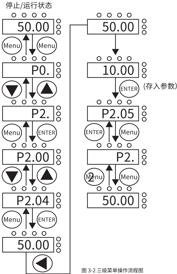
图 3-2 三级菜单操作流程图
