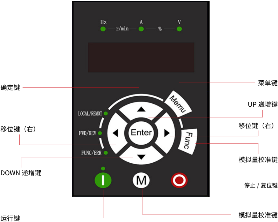
图 3-1 面板示意图
